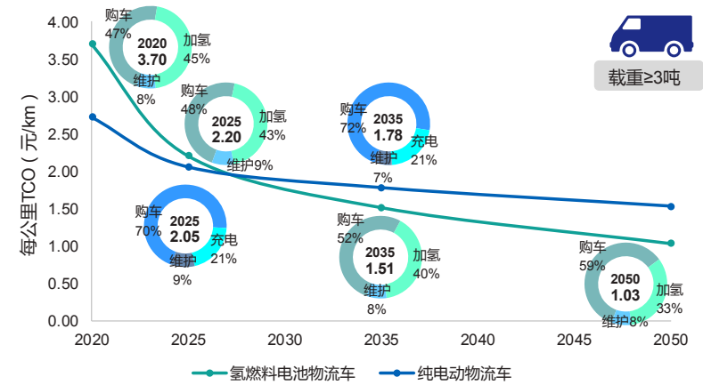
图表 5-5 氢燃料电池物流车的 TCO 成本经济性趋势
