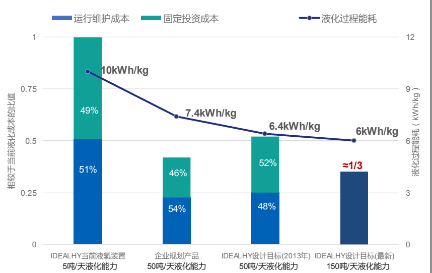
图表 5-28 IDEALHY 对未来氢液化能耗和成本的预期 64
