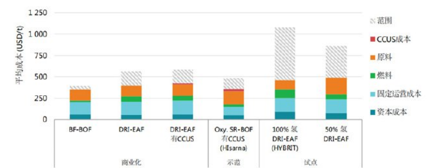
图表 5-18 不同钢铁生产工艺的吨钢成本及构成分析
