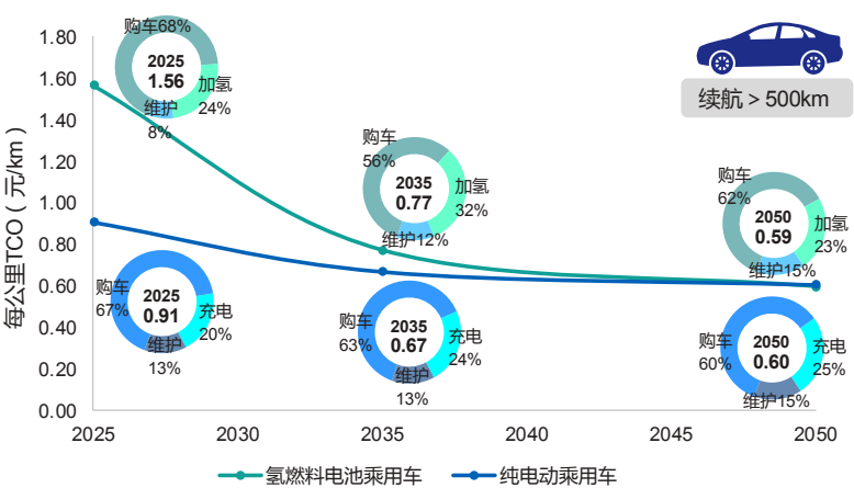
图表 5-9 氢燃料电池乘用车的 TCO 成本经济性趋势
