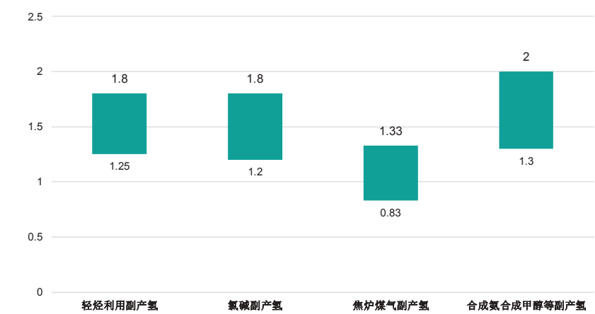
图表 3-6 中国工业副产氢制氢综合成本（元/Nm 3 ）
