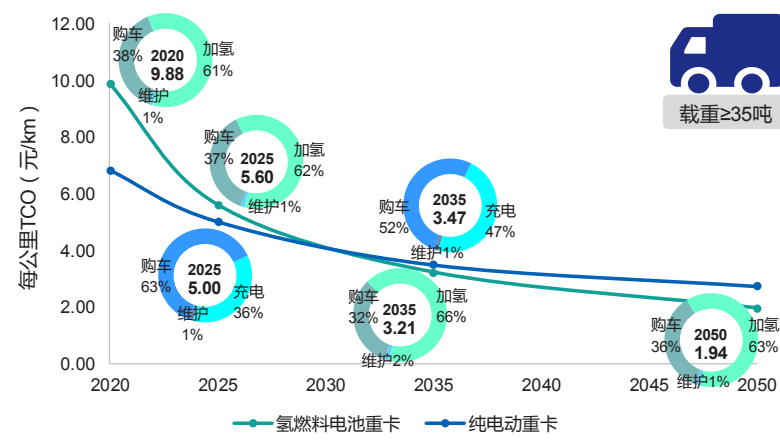
图表 5-7 氢燃料电池重卡的 TCO 成本经济性趋势
