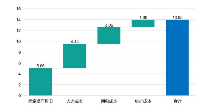
图表 6-5 加氢站运营成本折算到氢气销售量的价格（元/kg）
