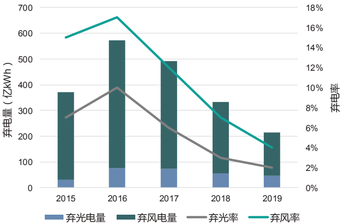
图表 5-14 我国弃风弃光现象存在
